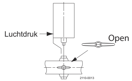
A/A actuator
