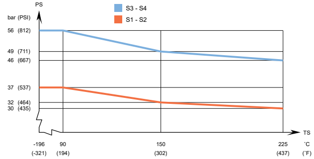
经 ACK73 - PED 认证的压力/温度曲线图
