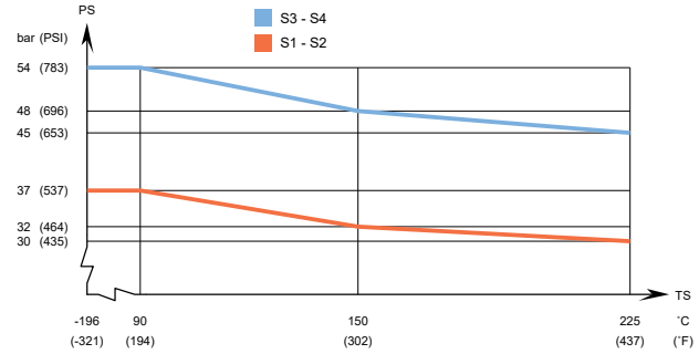
经 ACH73 - PED 认证的压力/温度曲线图
