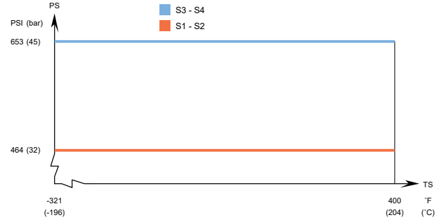
经 ACH73 - UL 认证的压力/温度曲线图
