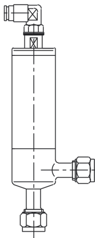
气动角阀
