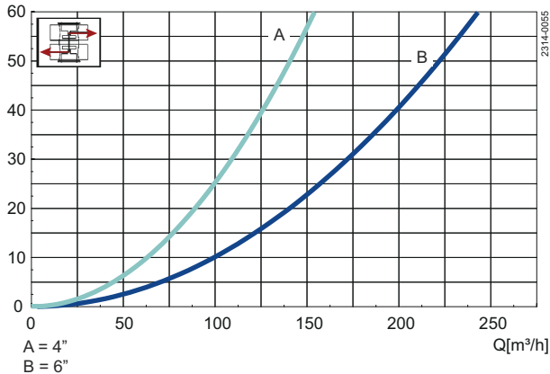
Abbildung 2. Druckabfall-/Leistungsdiagramm, zwischen den Gehäusen
