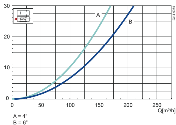
Abbildung 3. Druckabfall-/Leistungsdiagramm, unteres Gehäuse
