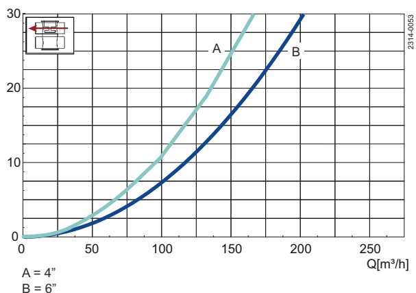
Abbildung 1. Druckabfall-/Leistungsdiagramm, obere Gehäuse
