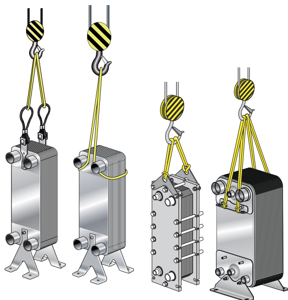
図 2 吊り上げ例。
