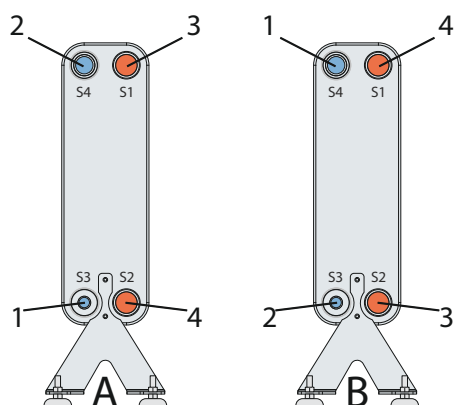
図 5 シングルサーキット式熱交換器 A 蒸発器、B 凝縮器。1.冷媒入口、2.冷媒出口、3.水/ブライン入口、4.水/ブライン出口
