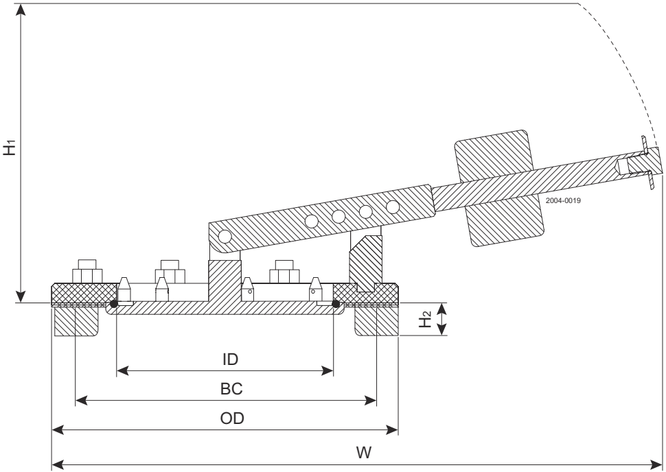
図 2. バルブを備えたフランジ
