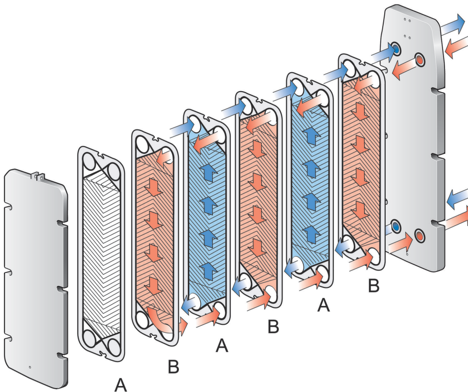
Figura 4: Principiul de aranjare a pachetului de plăci, cu garniturile îndreptate spre placa de presiune.
