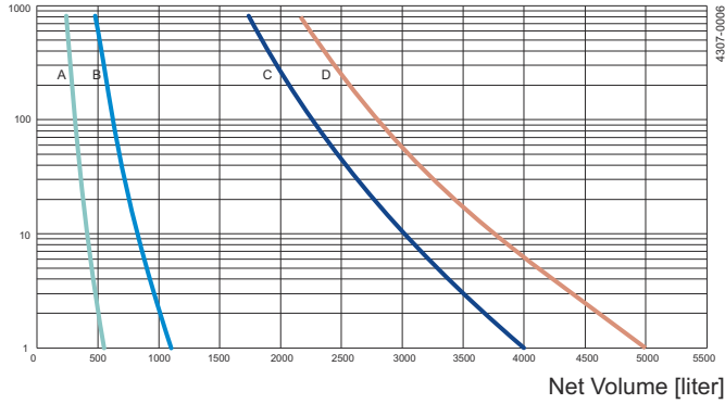
Abbildung 5. Leistungsstufe 3: Mischen Volumen vs. Viskosität
