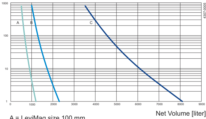
Abbildung 4. Leistungsstufe 2: Mildes Mischen Volumen vs. Viskosität
