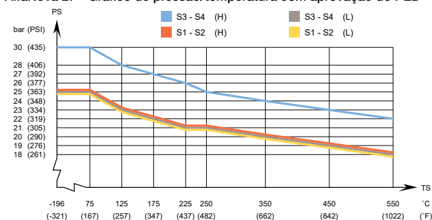
AlfaNova 27 - Gráfico de pressão/temperatura com aprovação do PED
