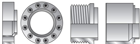
Kompaktní příruba
