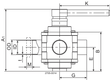
图 1. 带手柄的 MH53
