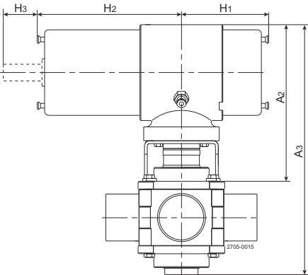
图 2. 带执行机构的 MH53, KH631 型
