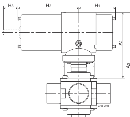
Figura 2. MH53 com atuador, tipo KH631
