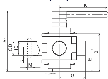
Figura 1. MH53 com manípulo
