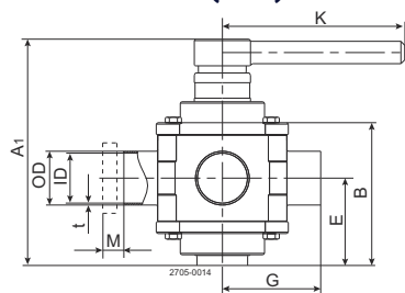
Figura 1. MH53 con mango
