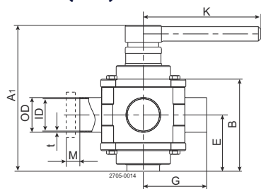
Abbildung 1. MH53 mit Griff
