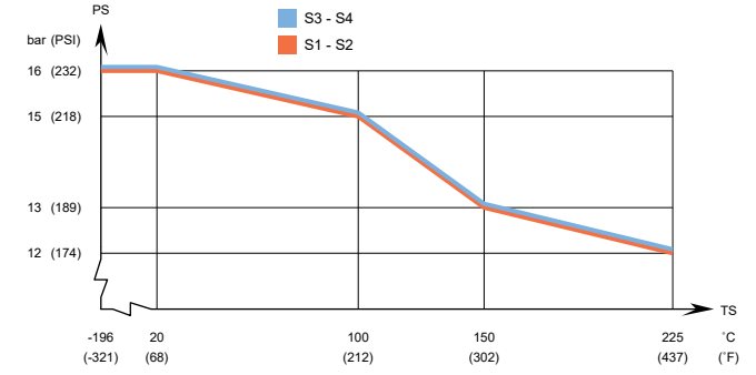
CB410 - PED 인증 압력/온도 그래프
