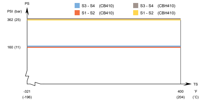
CB410/CBH410 - UL 인증 압력/온도 그래프
