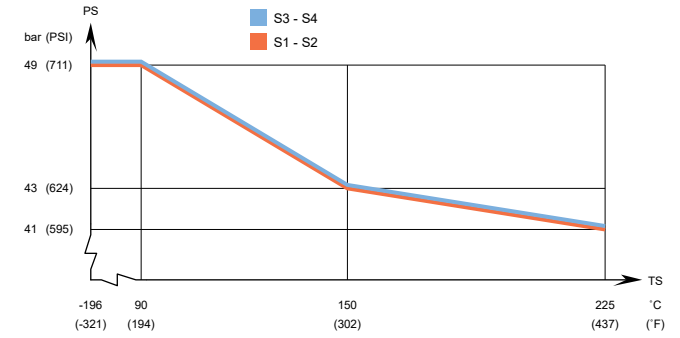
CBK410 - PED 인증 압력/온도 그래프
