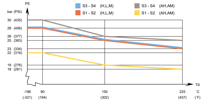
CBH410 - PED 인증 압력/온도 그래프
