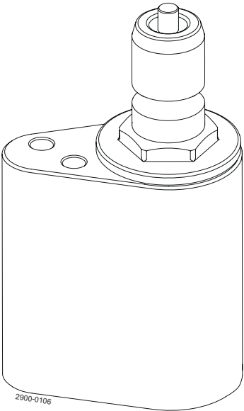
带止回阀的外螺纹快速接头
