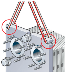
Figura 6: Elevación de los modelos AQ1, AQ2, AQ4, AQ1A, AQ2A, AQ2S, AQ1L y una versión anterior de los modelos AQ3, AQ2L
