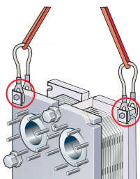
Figura 9: Elevación de los modelos AQ4T, AQ2T, AQ3, AQ2L
