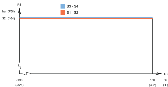
ACH502EQ - PED 許容圧力/温度グラフ
