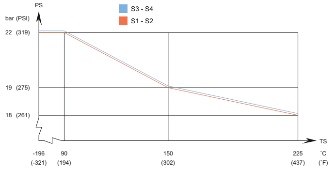
DOC410 - PED 인증 압력/온도 그래프
