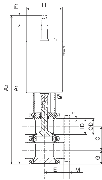
Direkt wirkendes Absperrventil
