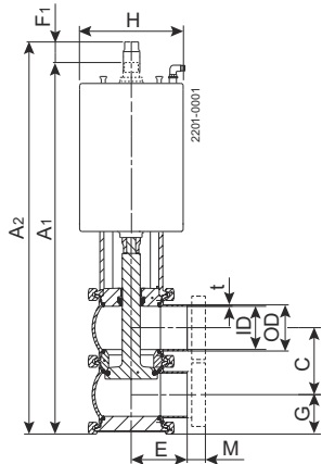
Rückwärts wirkendes Absperrventil
