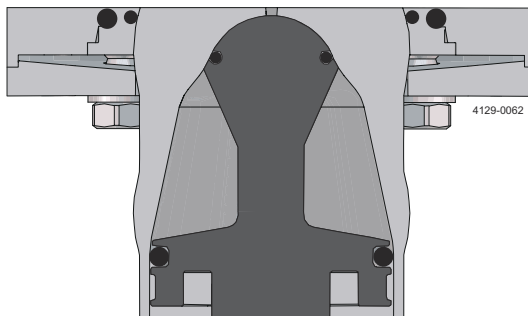
固定焊接板
