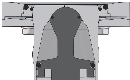
可调焊接板
