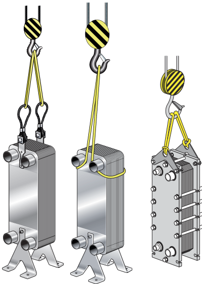
Figuur 2: Voorbeelden van hijsen.
