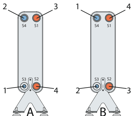
Figuur 5: Enkel circuit: A verdamper; B condensor. 1.Koudemiddelinaat 2.Koudemiddeluitlaat 3.Water/Brine inlaat 4.Water/Brine uitlaat
