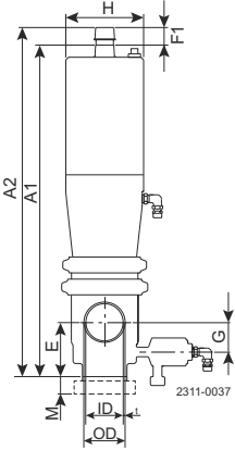
图 1. a. 截止阀
