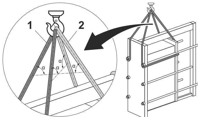
Figure 2 : L'illustration indique le filetage des élingues fixées sur un équipement utilisé pour l'exemple.
