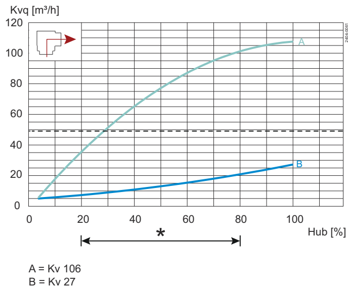
Abbildung 5. Ventilgröße ISO 2,5"/DN65
