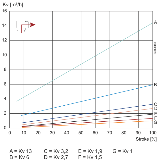
Abbildung 1. Ventilgröße ISO 1 Zoll
