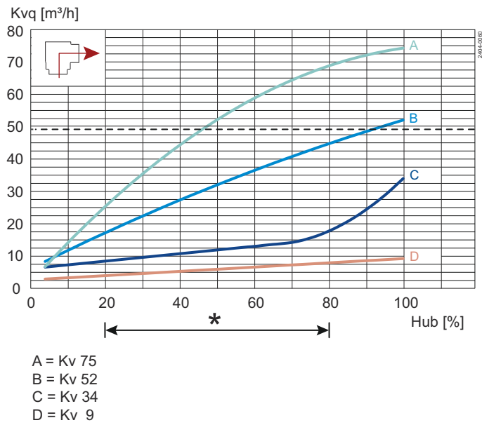
Abbildung 4. Ventilgröße ISO 2"/DN50
