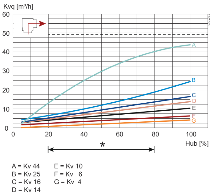
Abbildung 3. Ventilgröße ISO 1,5"/DN40
