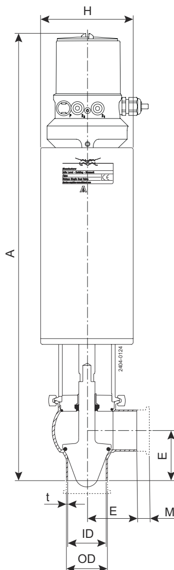
Abbildung 9. RV-ST-Ventil
