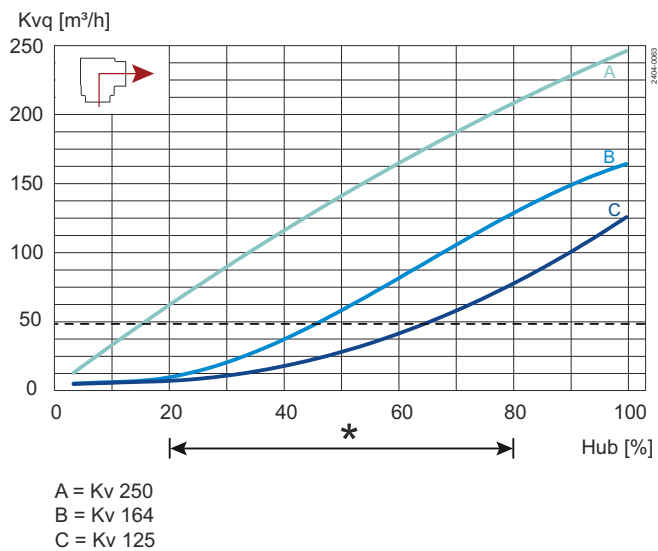
Abbildung 7. Ventilgröße ISO 4"/DN100
