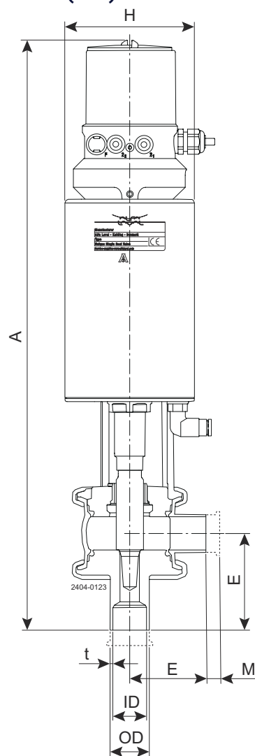
Abbildung 8. Nadelventil
