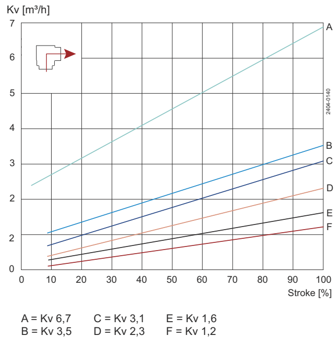
Abbildung 2. Ventilgröße (DN25)
