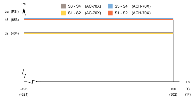
经 AC70X/ACH70X - PED 认证的压力/温度曲线图
