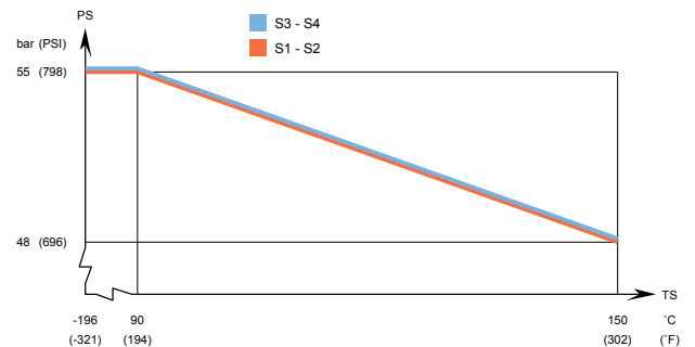
经 ACP70X - PED 认证的压力/温度曲线图
