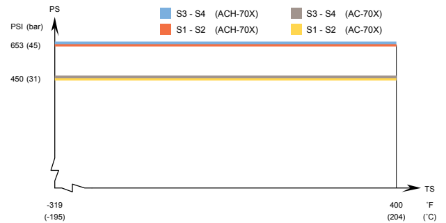
经 AC70X/ACH70X - UL 认证的压力/温度曲线图
