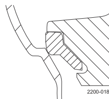
Figura 3. TR2-PTFE y TR3-PEEK Junta de tapón flotante
