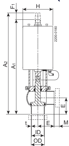
Figura 1. Válvula de cierre
