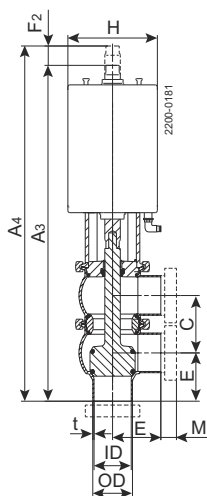
Figura 2. Válvula de desvío
