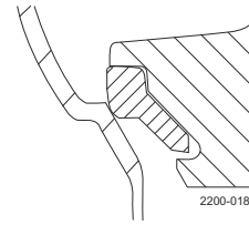
Abbildung 3. TR2-PTFE und TR3-PEEK Schwimmende Dichtung
