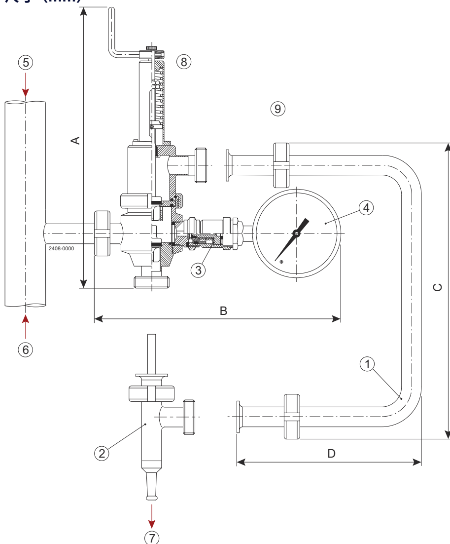
尺寸 (mm)
