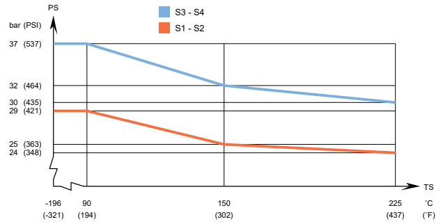
CB24 - PED 인증 압력/온도 그래프
