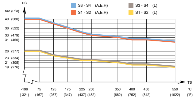
AlfaNova HP 76 - PED 인증 압력/온도 그래프 1
