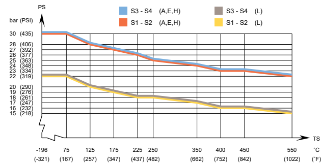
AlfaNova 76 - PED 인증 압력/온도 그래프 1
